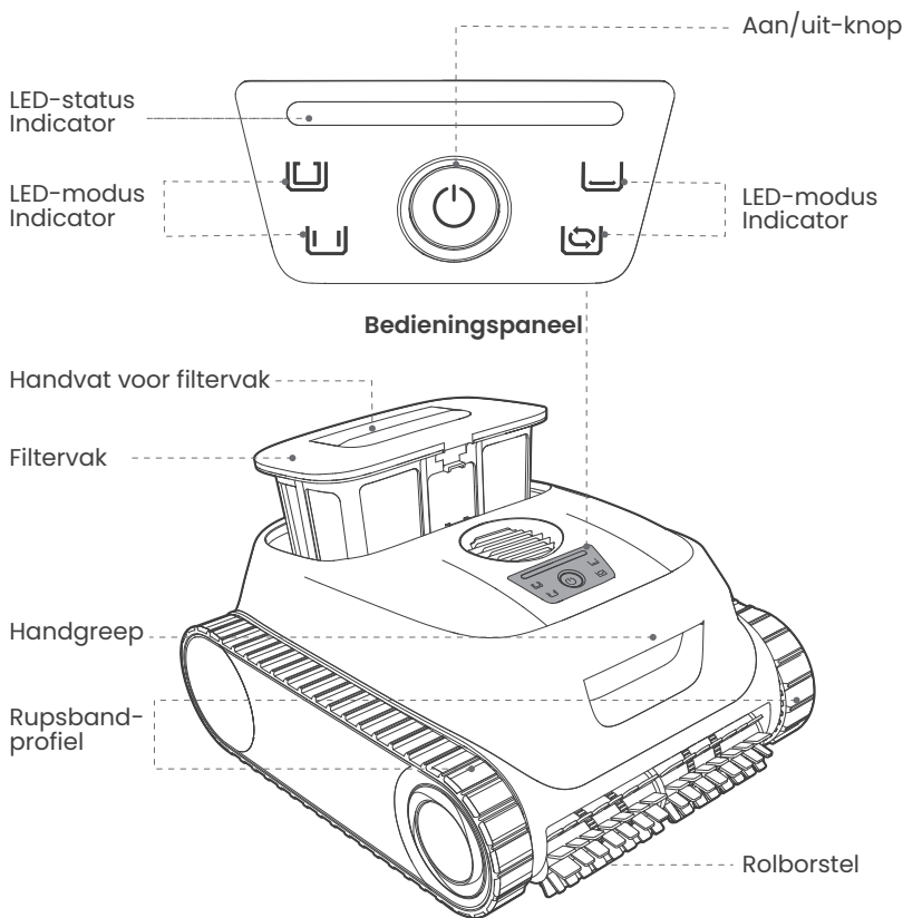
Robot voor zwembadreiniging (zijaanzicht)
