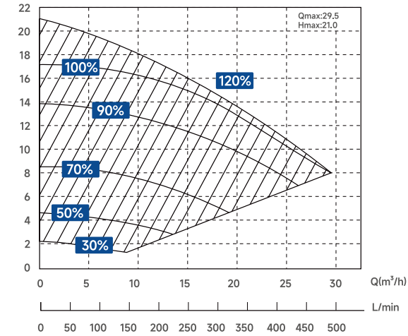
H(m) IP30
