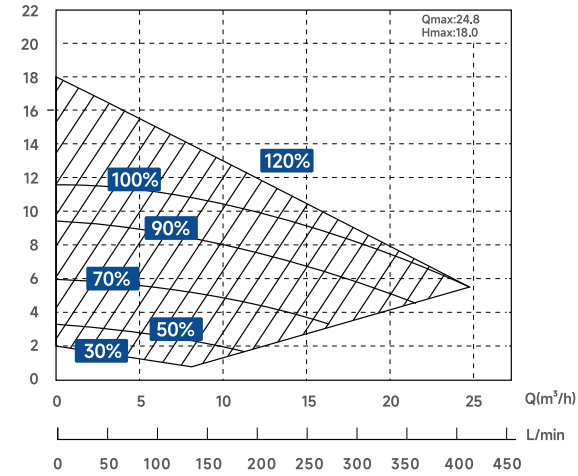
H(m) IP20
