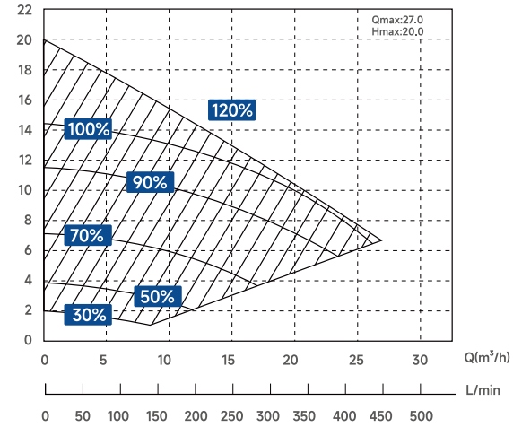
H(m) IP25
