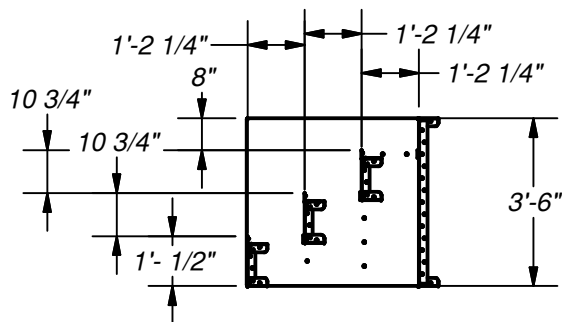
SECTION A-A SCALE .25:12
