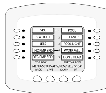
iS10 circuit/button setup
