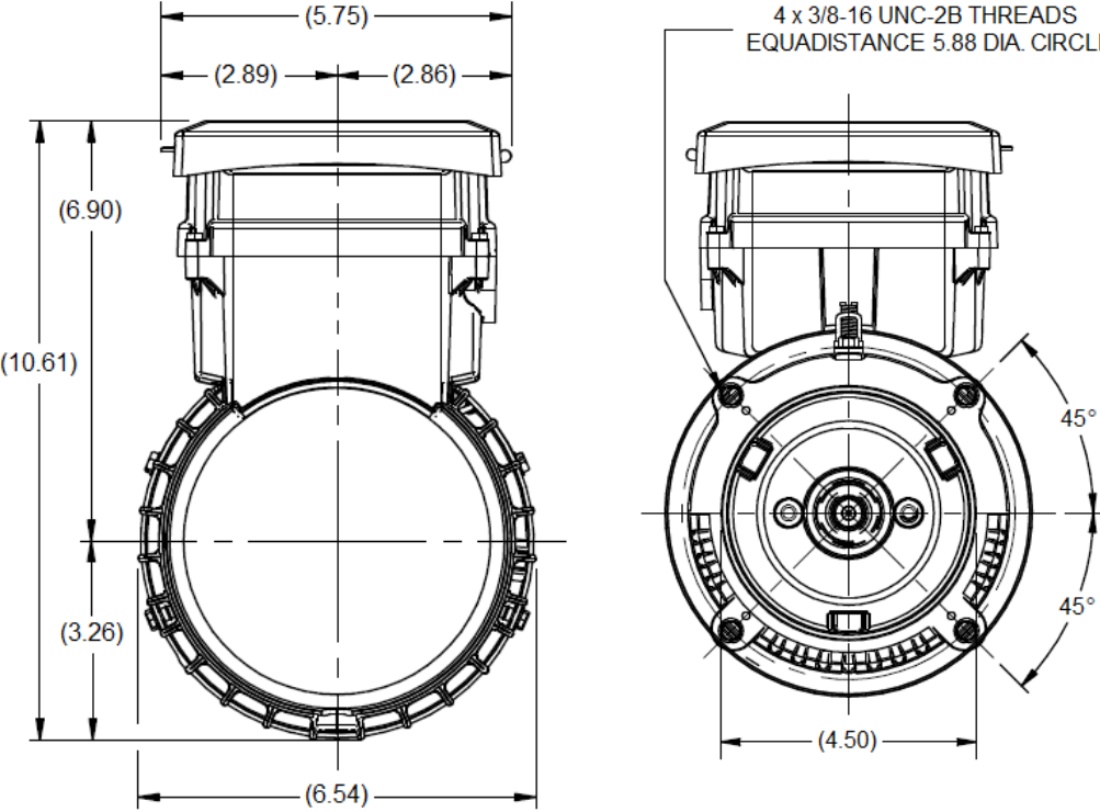
Fan View
