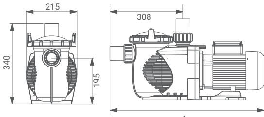
Côte «A» = 652mm sauf 682mm pour EMX-100-0016
