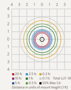
RW 9LED ISOFOOTCANDLE PLOT
