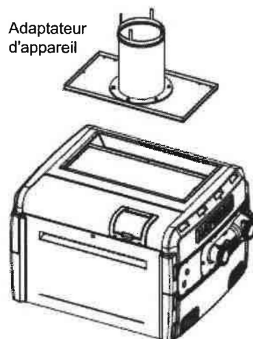
Figure5 Installer l'adaptateur
