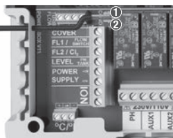
Sensor geleidbaarheid ① geel ② doorzichtig
