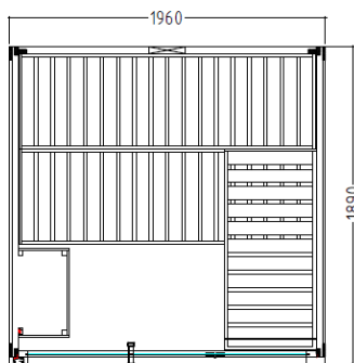
Installation en miroir possible (banquette côté poêle)
