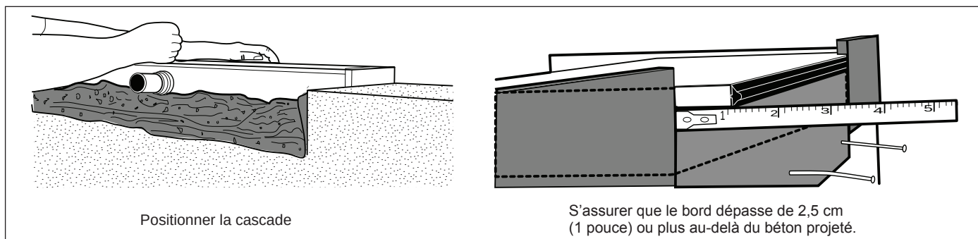
Figure 7. Positionnement de la cascade dans l'encoche
