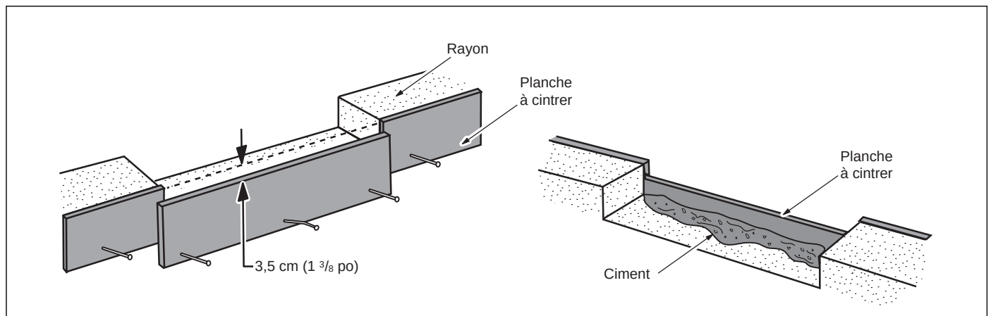
Figure 5. Installer la planche à cintre
