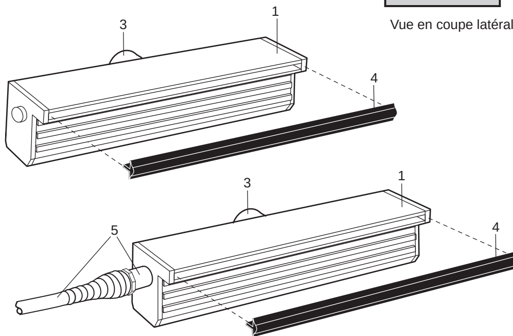
Figure 2. Composants des cascades Sheer Descent et FiberFall
