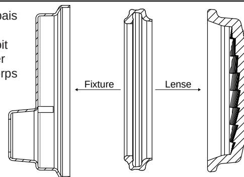
Illustration 10. Vue en coupe de la lampe à DEL WaterColors Pro Series de Jandy
