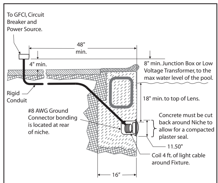
Figura 1. Instalación de la luz de colores digital Jandy Pro Series
