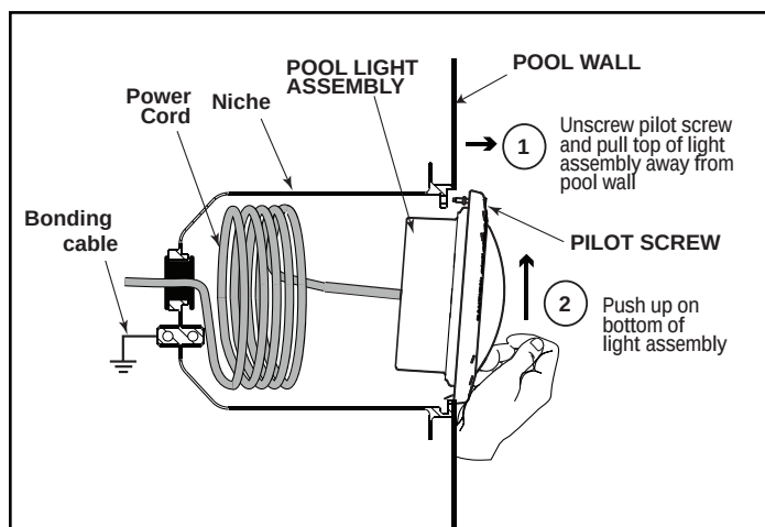
Illustration 6. Démontage de la lampe à DEL RGBW WaterColors Pro Series de Jandy pour remplacer le moteur de la lampe
