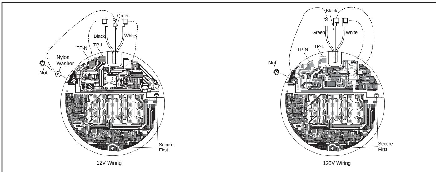
Figura 8. Reemplazo y cableado del motor (PCB) de luz grande
