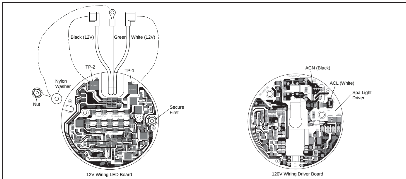
Figura 7. Reemplazo y cableado del motor (PCB) de luz pequeña
