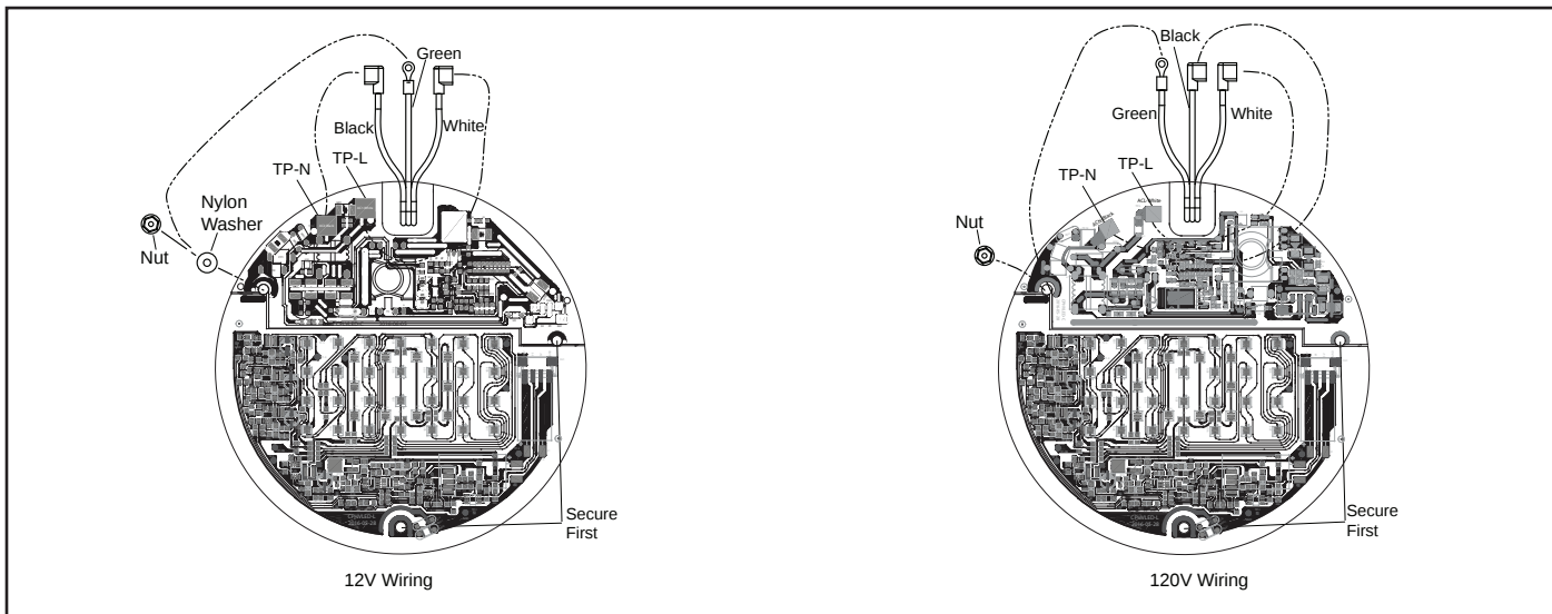
Illustration 8. Remplacement et câblage du moteur de la grande lampe (carte de circuits imprimés)
