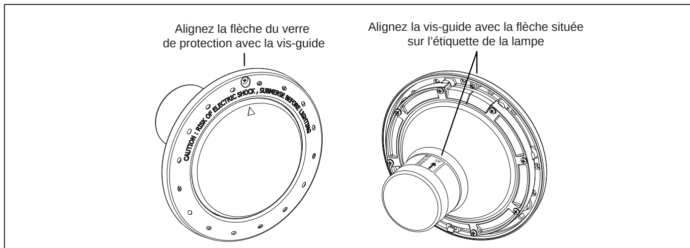
Figure 2. Alignement du verre de protection, de la bague avant, du boîtier et des crochets supports des lampes blanches de piscine
