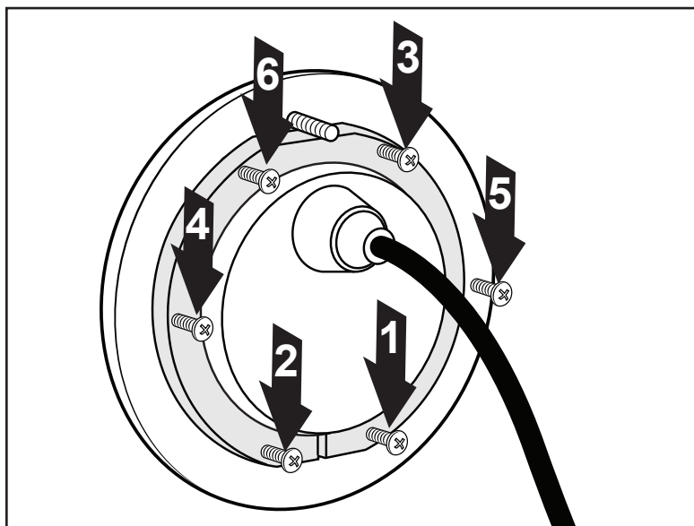
Figura 6 Apriete los tornillos en un patrón de estrella
