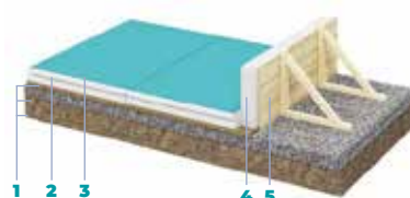
Étape 3 1 Support compacté 2 Panneaux THERMAPOOL SSD (selon épaisseur) 3 Film polyéthylène selon nécessité chantier 4 Planelle découpée au sein d'un panneau THERMAPOOL (hauteur = épaisseur THERMAPOOL + épaisseur dalle + 100 mm) 5 Coffrage
