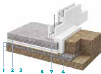
Étape 5 1 Support compacté 2 Panneaux THERMAPOOL SSD 3 Film polyéthylène selon nécessité chantier 4 Planelle découpée au sein d'un panneau THERMAPOOL (hauteur = épaisseur THERMAPOOL + épaisseur dalle + 100 mm) 5 Coffrage 6 Béton armé (selon les préconisations de l'étude de conception) 7 Blocs coffrants (blocs dédiés piscine en polystyrène expansé ou alternative adaptée)
