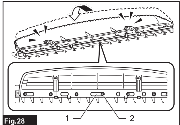
► 1. Hole 2. Screw
