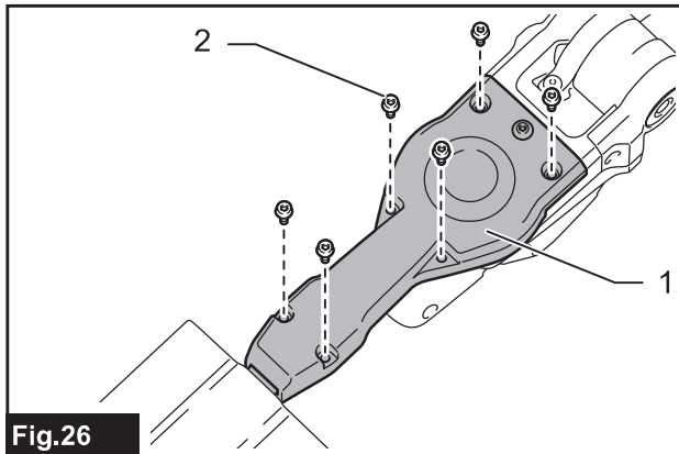
► 1. Cover 2. Bolt
