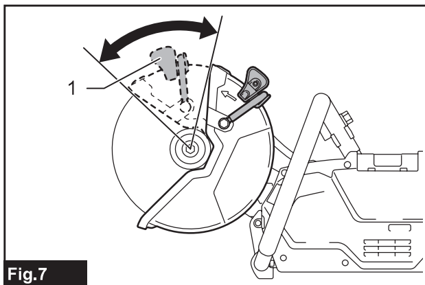
► 1. Empuñadura de la cubierta de la rueda
