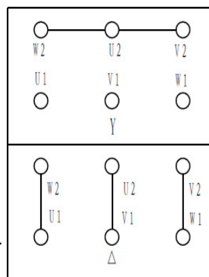
Dreiphasen-Schaltplan
