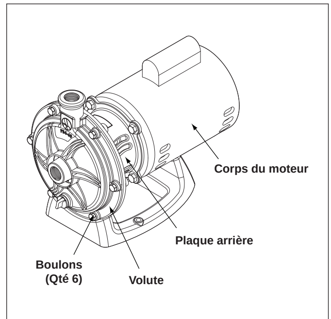
Figure 8. Retirer la volute de la pompe
