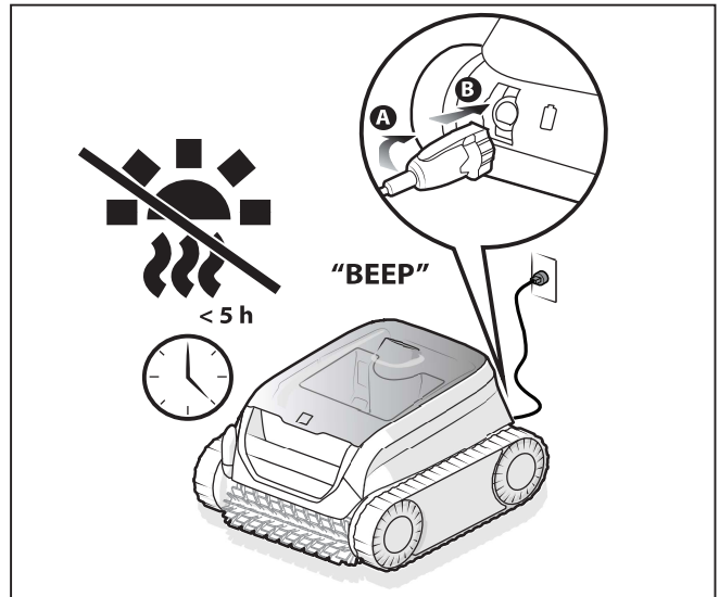
Figure 3. Connectez le nettoyeur et branchez-le
