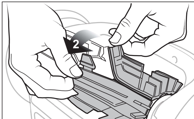
Figura 21. Desenganche las lengüetas del cepillo
