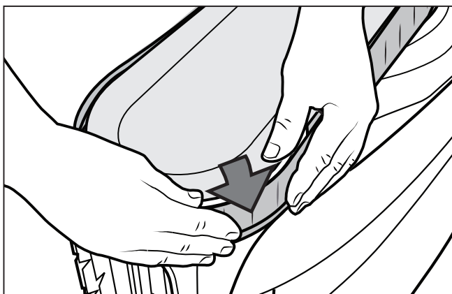
Figura 28. Comience por un lado de la oruga
