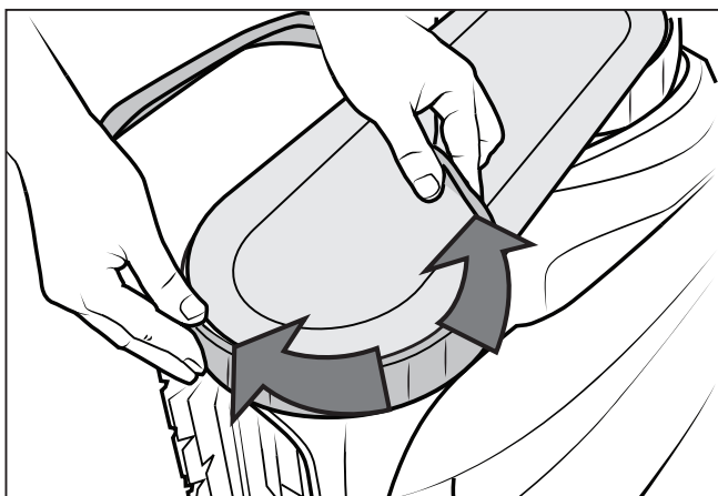
Figura 29. Acomode la oruga alrededor de la rueda
