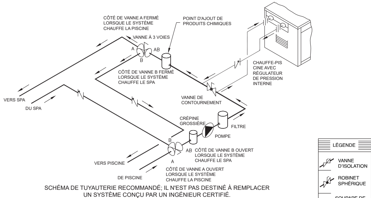
Figure 29. Installation, un seul appareil de chauffage
