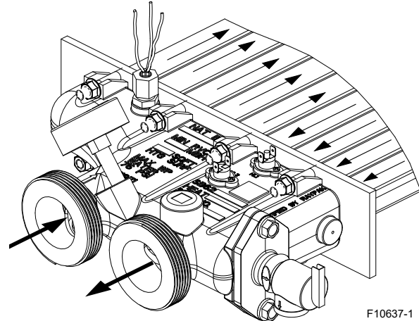
Figure 16. Débits d'eau, distributeur en bronze (ASME)
