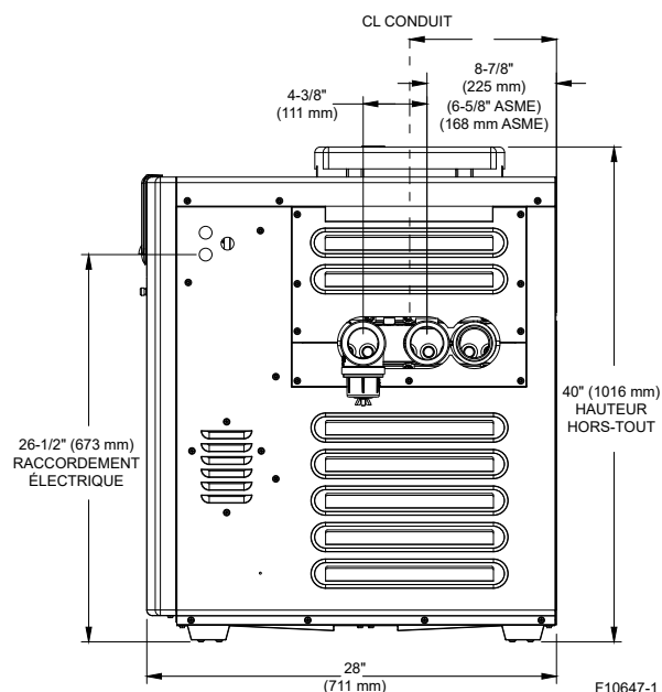
Figure 9. Vue de côté
