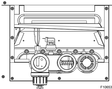
Figure 27. Raccords électriques, distributeur d'entrée/sortie
