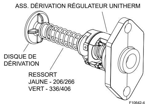
Figure 22. Vanne de dérivation automatique interne (ASME)
