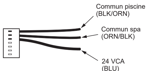
Figure 48. Harnais de câble à 7 broches pour thermostat externe
