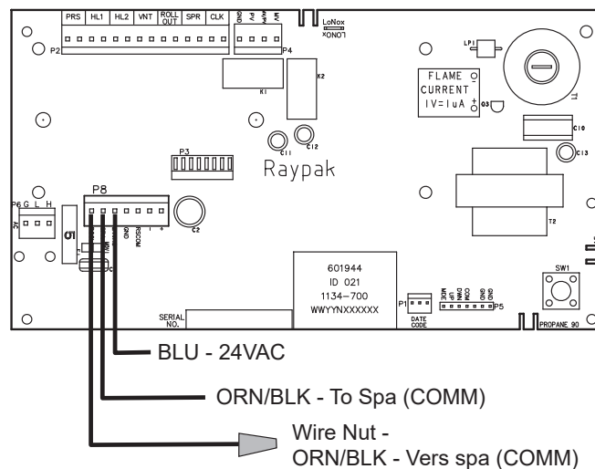
Figure 49. Connexion du harnais de câble d'un thermostat à 2 fils au connecteur P8
