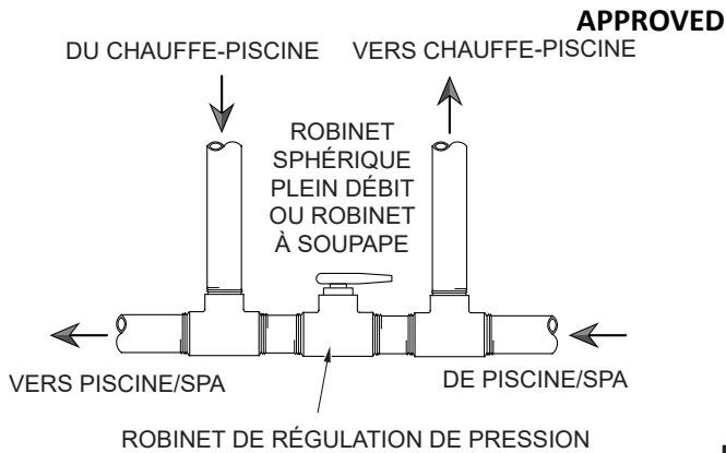
Figure 23. Vanne de dérivation auxiliaire
