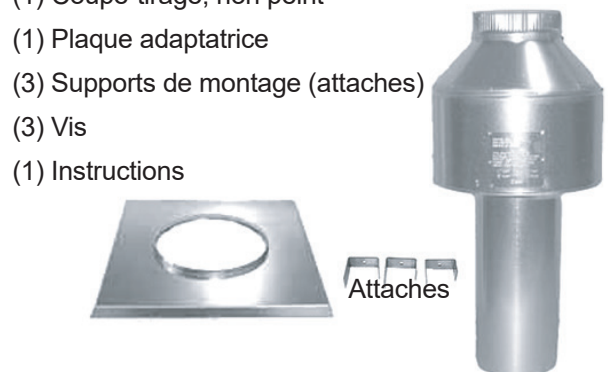
Figure 6. Composants, kit d'évacuation intérieur
