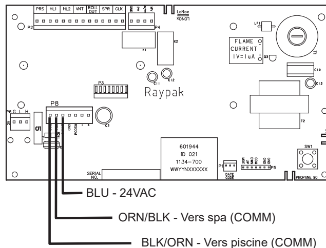
Figure 50. Connexion du harnais de câble d'un thermostat à 3 fils au connecteur P8
