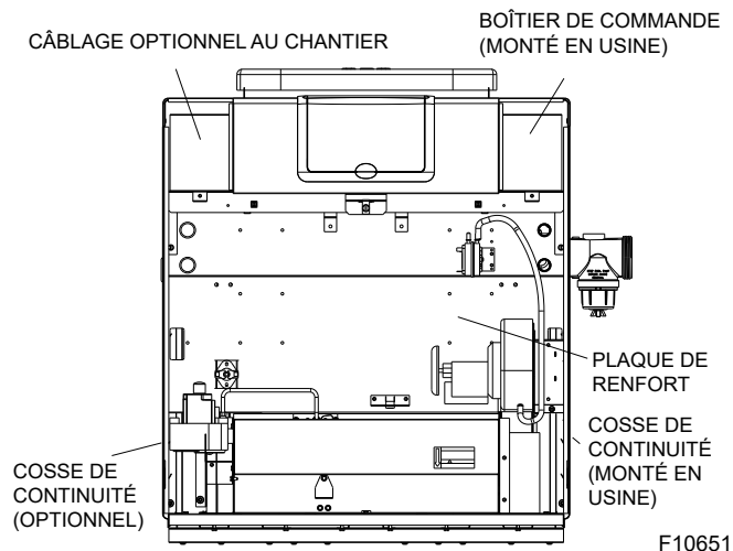
Figure 31. Emplacement du câblage
