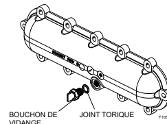
Figure 63. Bouchon de vidange du raccord de retour, modèles résidentiels (préfixe P)
