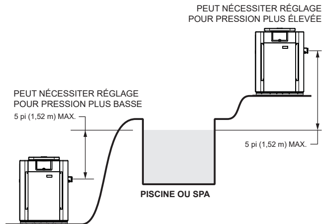
Figure 52. Configurations nécessitant un réglage
