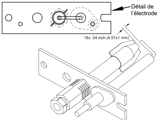
Figure 56. Veilleuse Lo NOx
