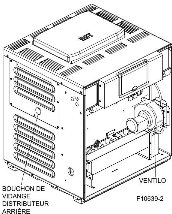
Figure 35. Emplacement des commandes (2)
