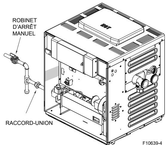
Figure 13. Installation du robinet d'arrêt manuel
