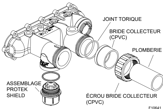
Figure 17. Distributeur d'entrée/sortie - polymère
