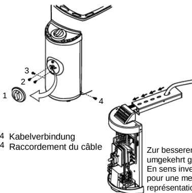
Abb. 3A Öffnen des Steuergeräts Fig. 3A Ouverture de l'unité de commande
