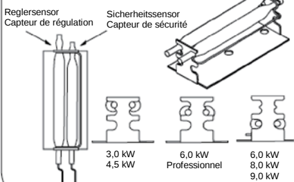
Abb. 10 | Anordnung der Sensoren Fig. 10 | Emplacement du capteur
