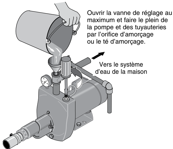
Figure 15 : Ouvrir la vanne de réglage
