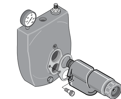
Figura 3: Monte el Eyector - Pozo Poco Profundo
