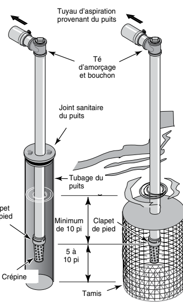
Figure 5 : Installations typiques dans un puits peu profond
