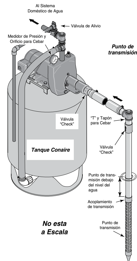
Figura 5: Instalación típica para pozo poco profundo
