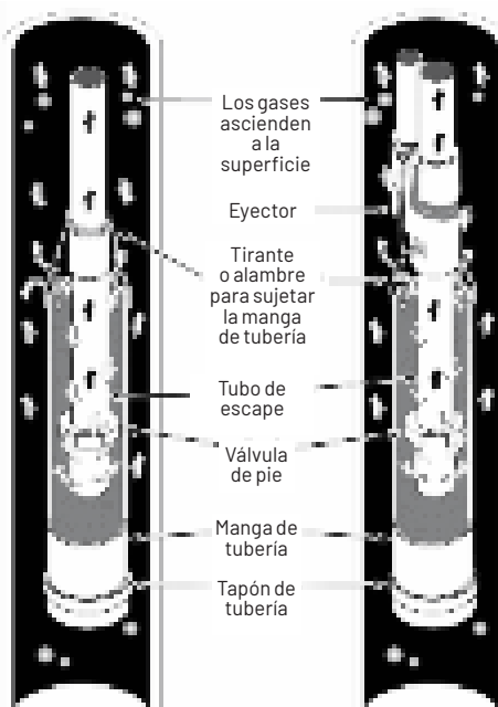
Figura 15: Control de gases/aire en el pozo
