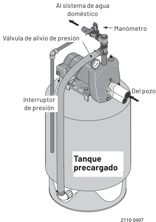
Figura 6: Conexiones de tanque precargado
