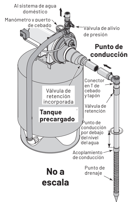
Figura 5: Instalaciones típicas de pozos poco profundos
