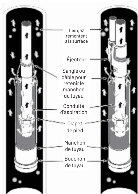
Figure 15 : Contrôle des gaz/de l'air dans le puits
