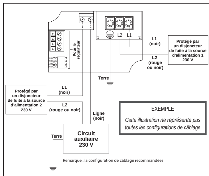
Figure 11. Schéma de câblage des sources d'alimentation distinctes de 230 V, de la charge auxiliaire
