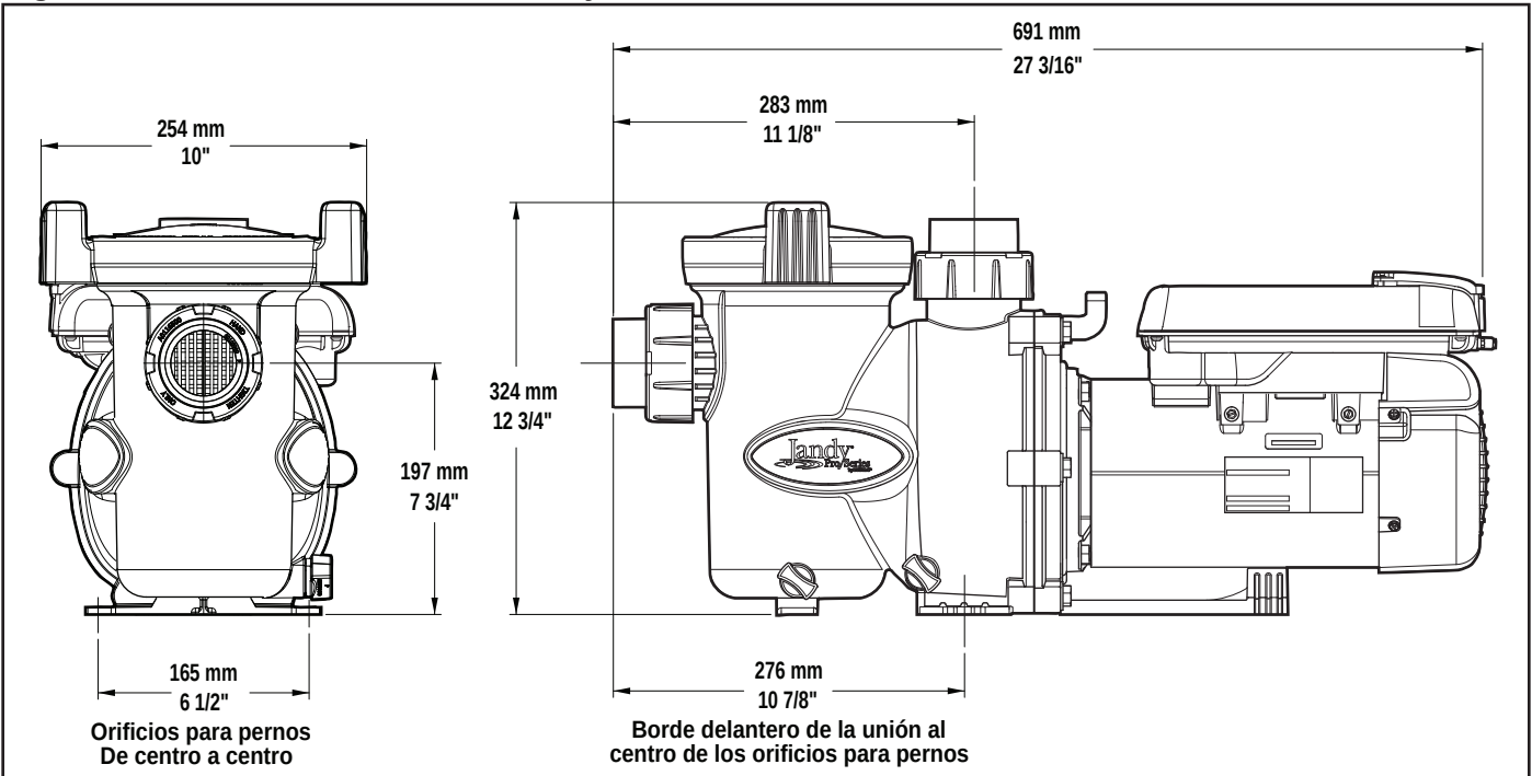
Figura 17. Dimensiones de la VS-FHP2.0 y VSFHP270AUT
