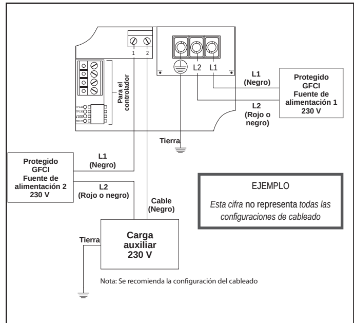
Figura 11. Diagrama de cableado de fuentes de alimentación separadas, carga auxiliar de 230 V
