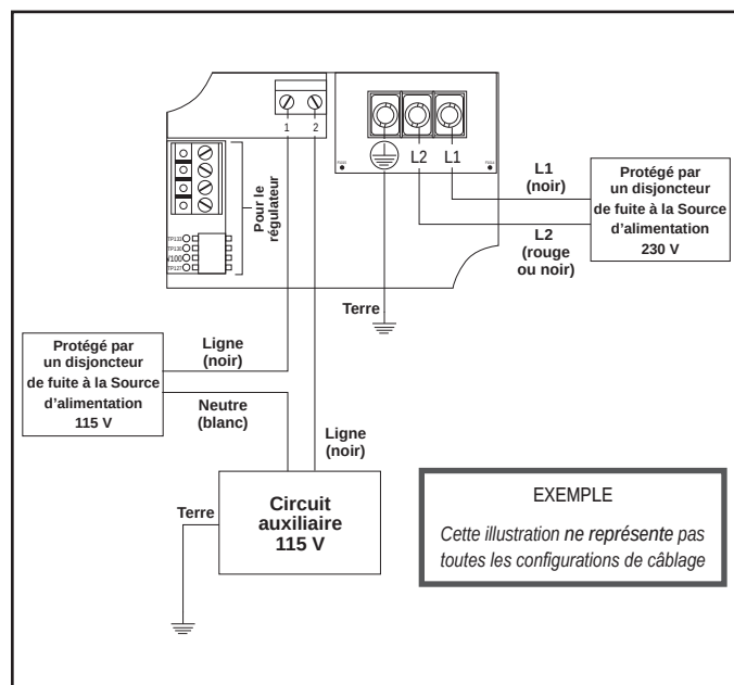
Figure 12. Schéma de câblage des sources d'alimentation partagées de 115 V, de la charge auxiliaire
