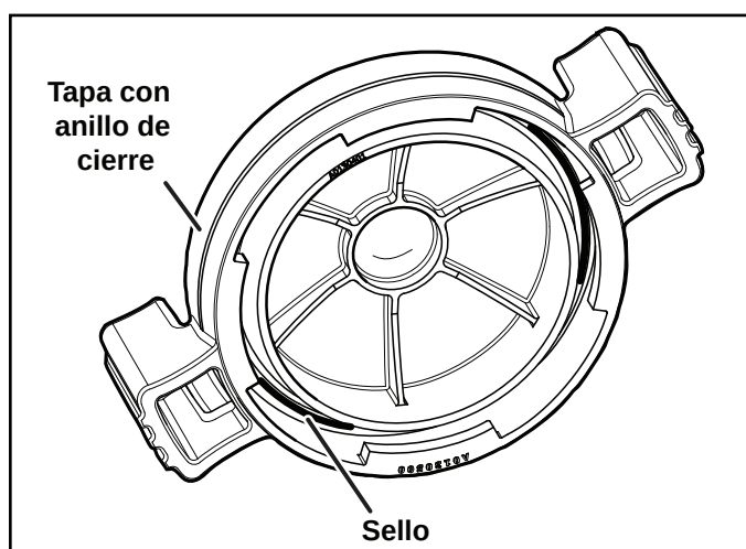
Figura 13. Anillo tórico en la tapa de montaje
