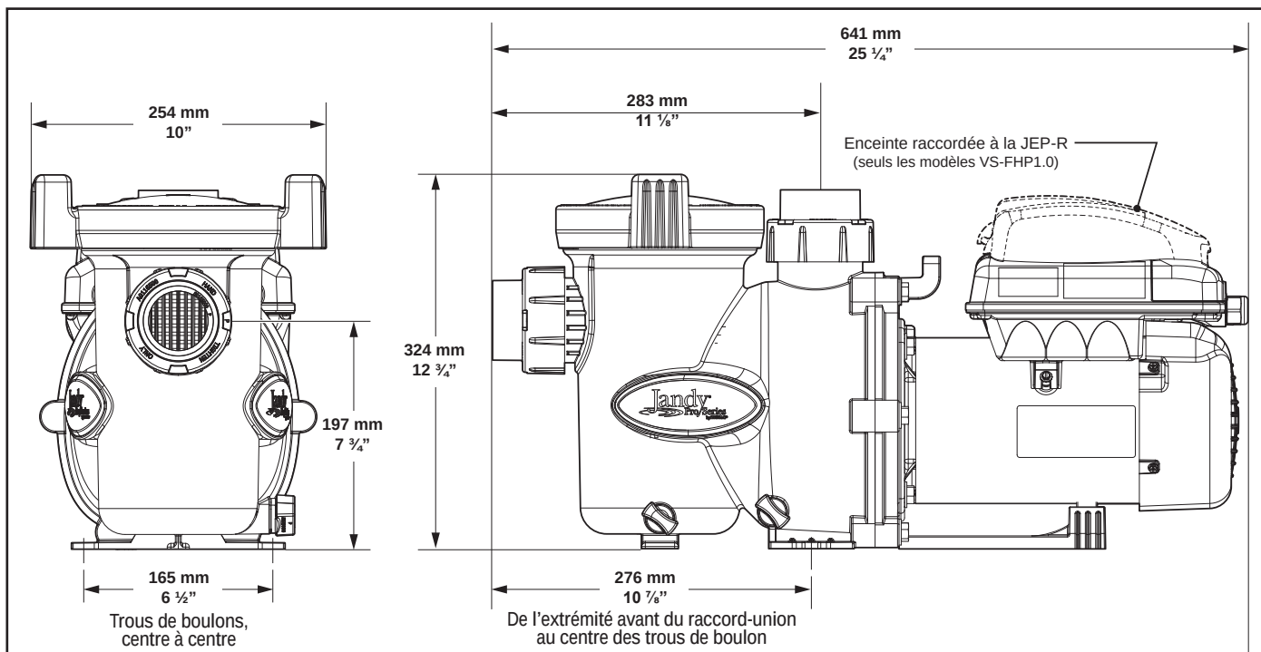
Figure 16. Dimensions de la VS-FHP1.0 et VSFHP165AUT
