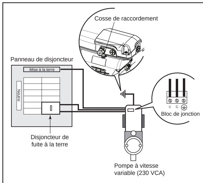
Figure 6. Raccordement du moteur
