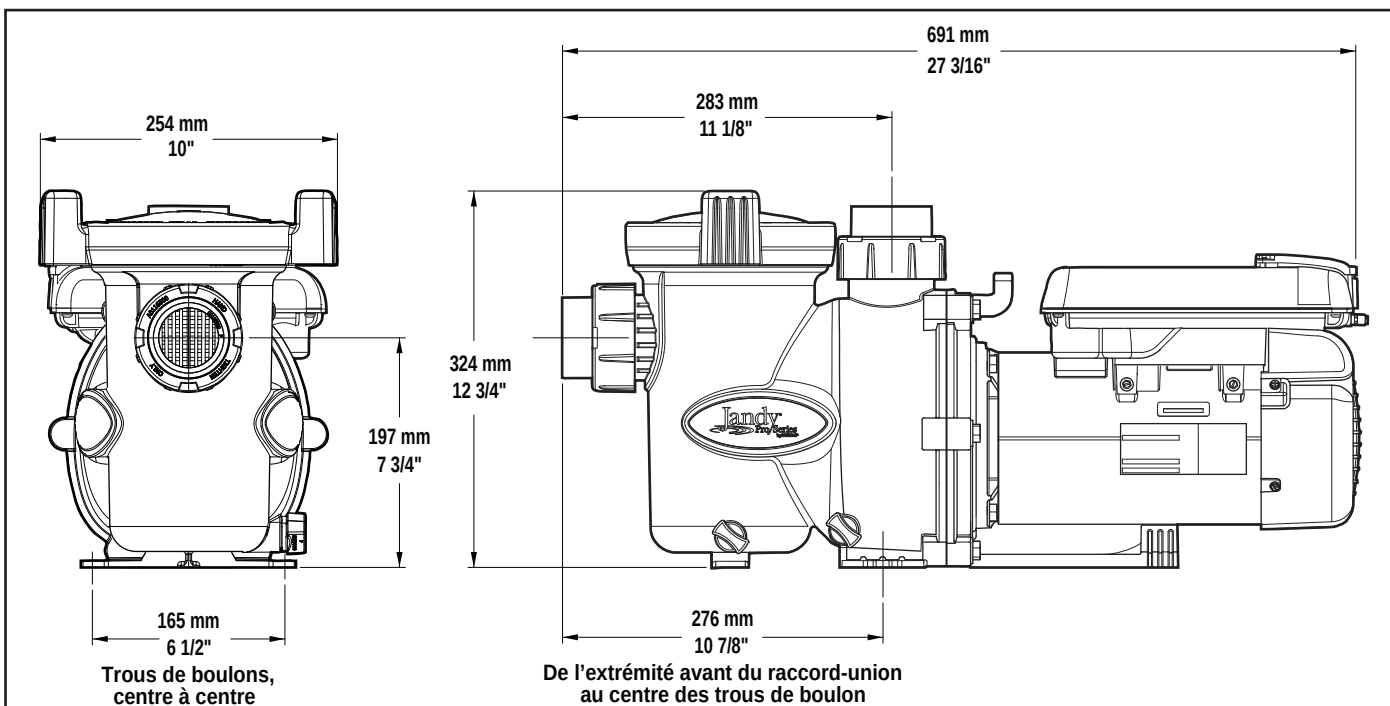
Figure 17. Dimensions de la VS-FHP2.0 et VSFHP270AUT
