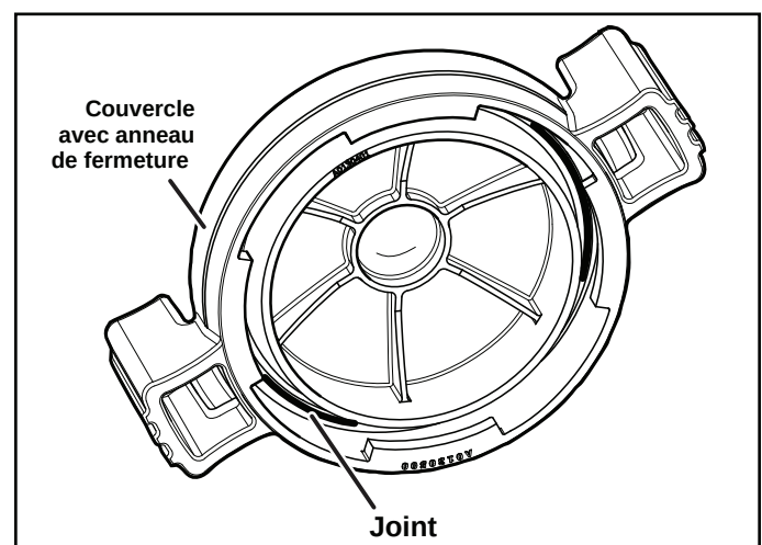
Figure 13. Joint torique dans l'ensemble couvercle
