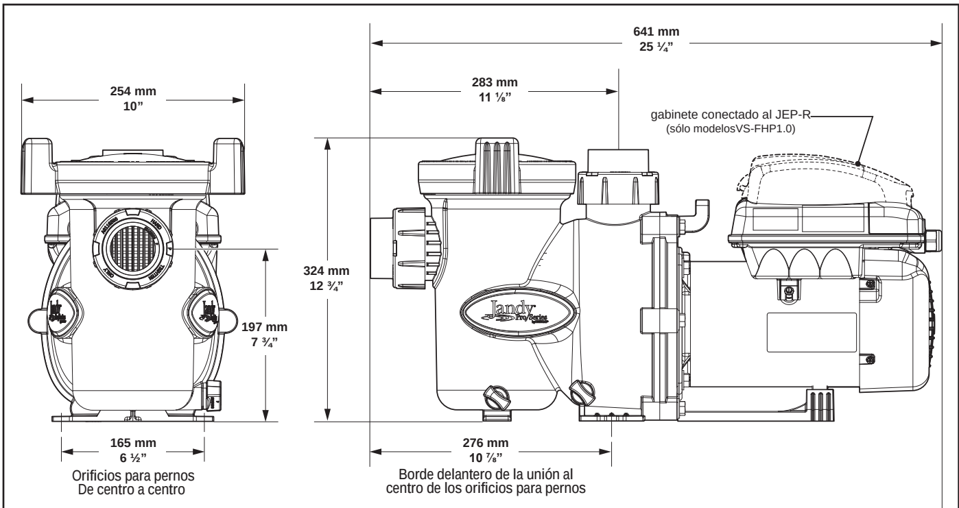
Figura 16. Dimensiones de la VS-FHP1.0 y VSFHP165AUT
