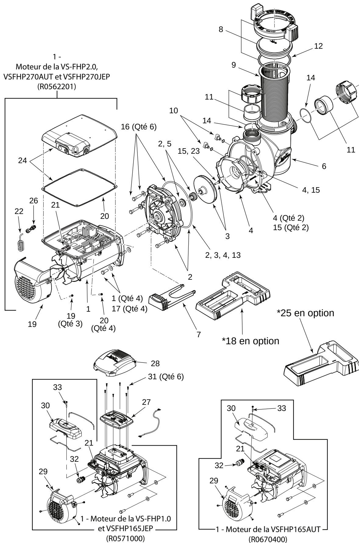
Figure 15. Vue éclatée des pompes de la série VS FloPro de Jandy
