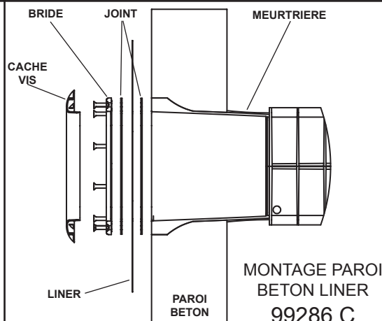
MONTAGE PAROI BETON
